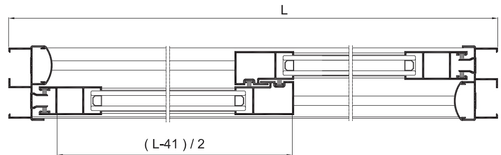
Sección A-A'
