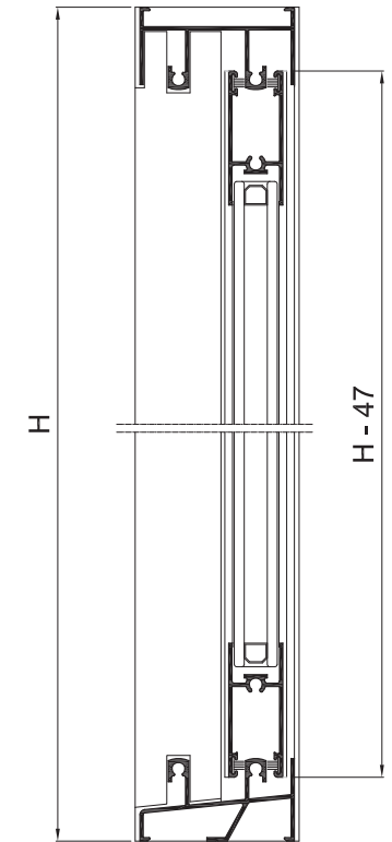
Sección B-B'
